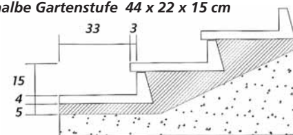
Gartenstufen ermöglichen den eleganten Aufbau von Treppen mit einem Unterschnitt
